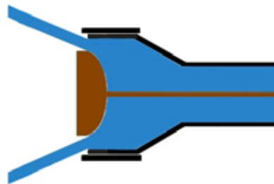
Bild 2: Umlenkkörper am Düsenaustritt erzeugt einen Sprühstrahl (schematische Darstellung)
