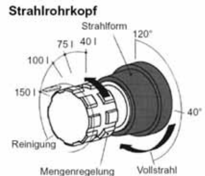
Bild 13: Bsp. für 4 Durchflussmengen u. Spülstellung am Stellring
